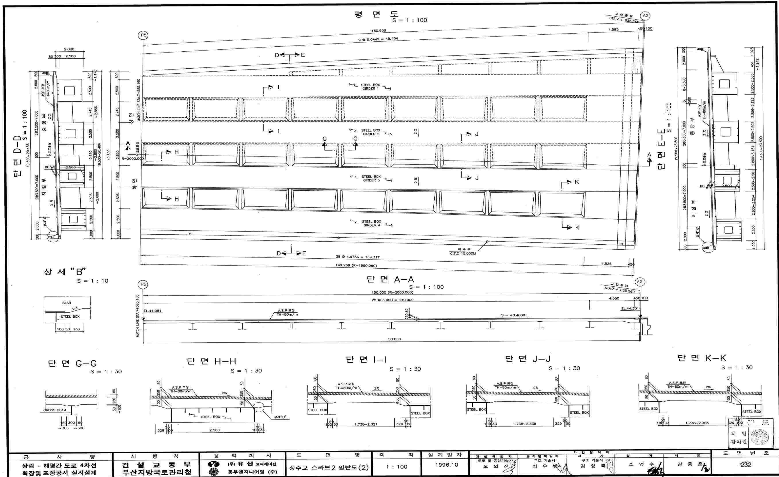
【그림 1.13】 슬라브 일반도(2)
