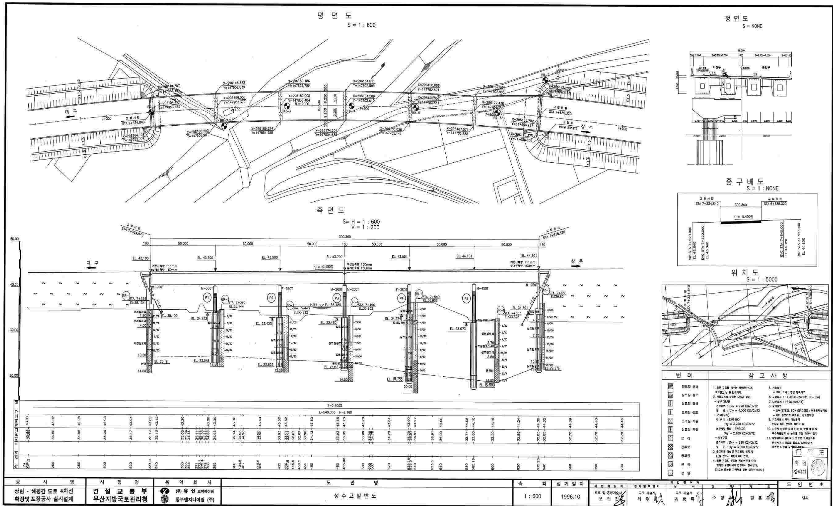
【그림 1.1】 교량 종평면도
